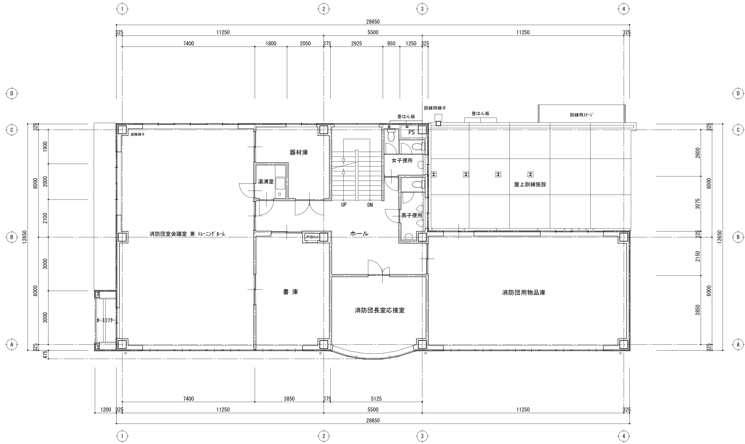
4階平面図 1/100
