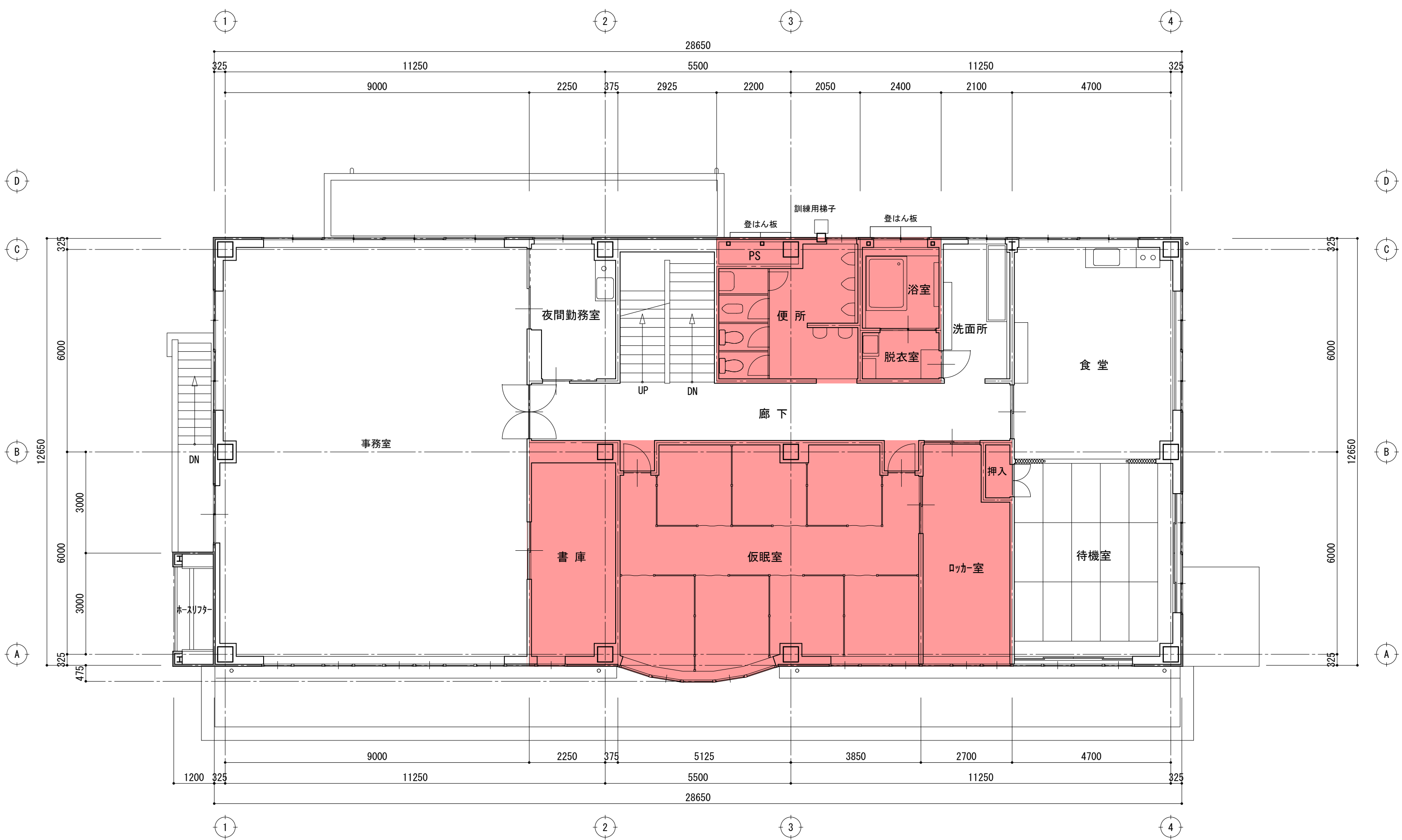
3階平面図 1/100
