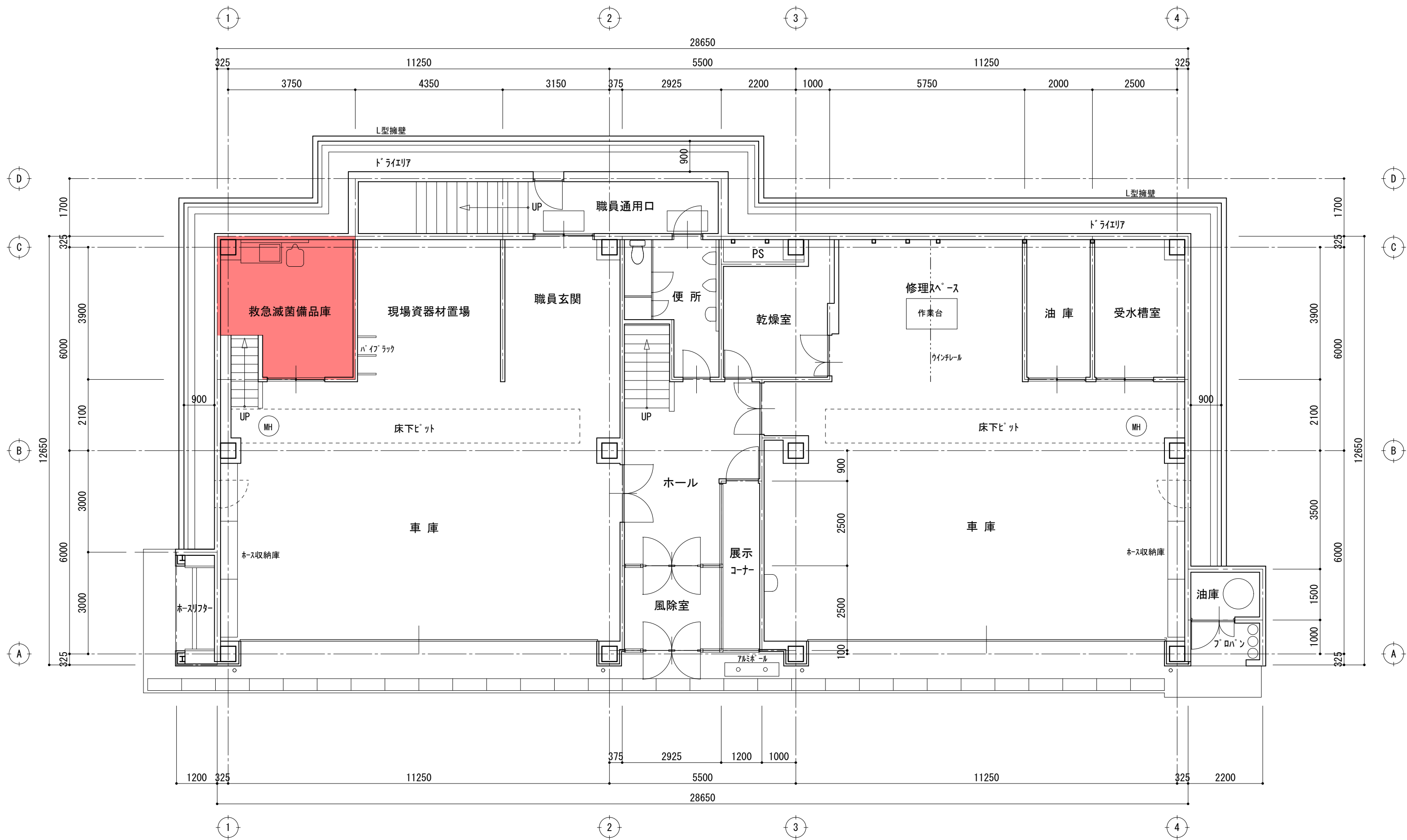
1階平面図 1/100
