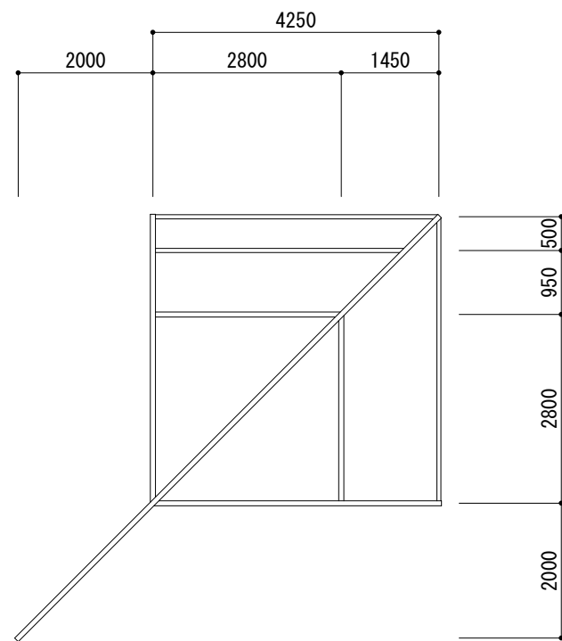
α-7° 結着用工作物平面図 1/100
